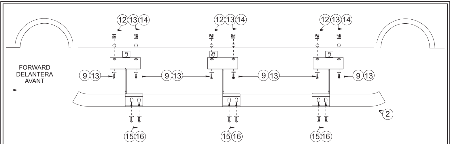
FIGURE 1 INSTALLATION VIEW OF DRIVER SIDE SHOWN, PASSENGER SIDE OPPOSITE FIGURA 1 VISTA DE LA INSTALACIÓN DEL LADO DEL CONDUCTOR OPUESTO AL LADO DEL ACOMPAÑANTE FIGURE 1 ILLUSTRE: COTE CONDUCTEUR, EN FACE: COTE PASSAGER
